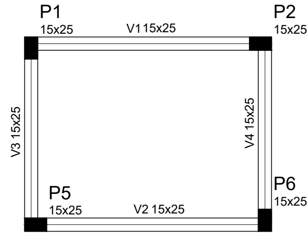
PLANTA DE FORMAS ESCALA S/E
